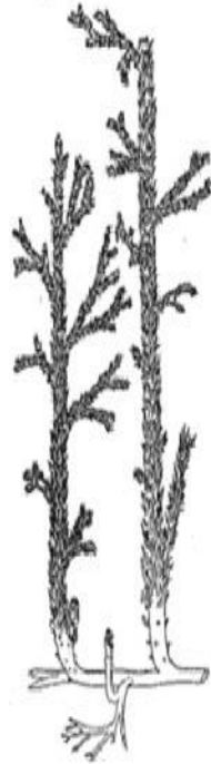
Астероксилон ( Asteroxylon )
